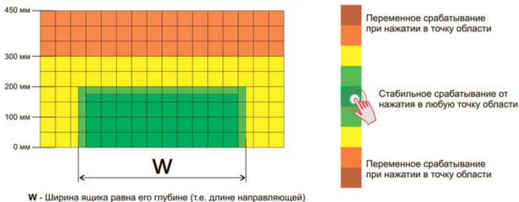
Область срабатывания механизма Push в зависимости от размеров фасада и габарита ящика
