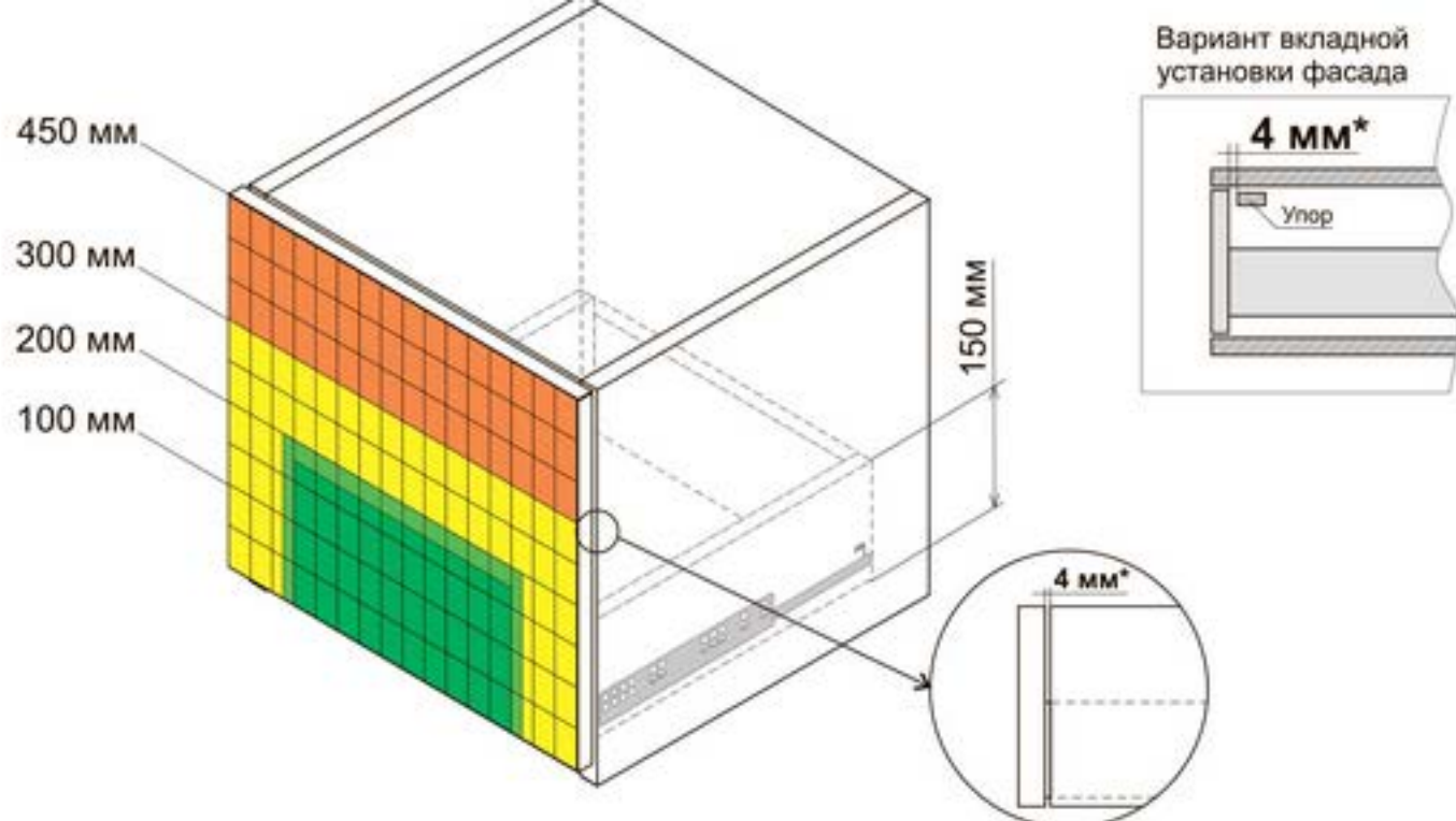
Область срабатывания механизма Push в зависимости от размеров фасада и габарита ящика
